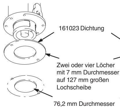
Montage mit 2 Bohrungen
