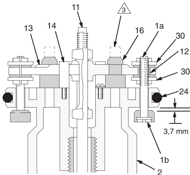
Schnittansicht
