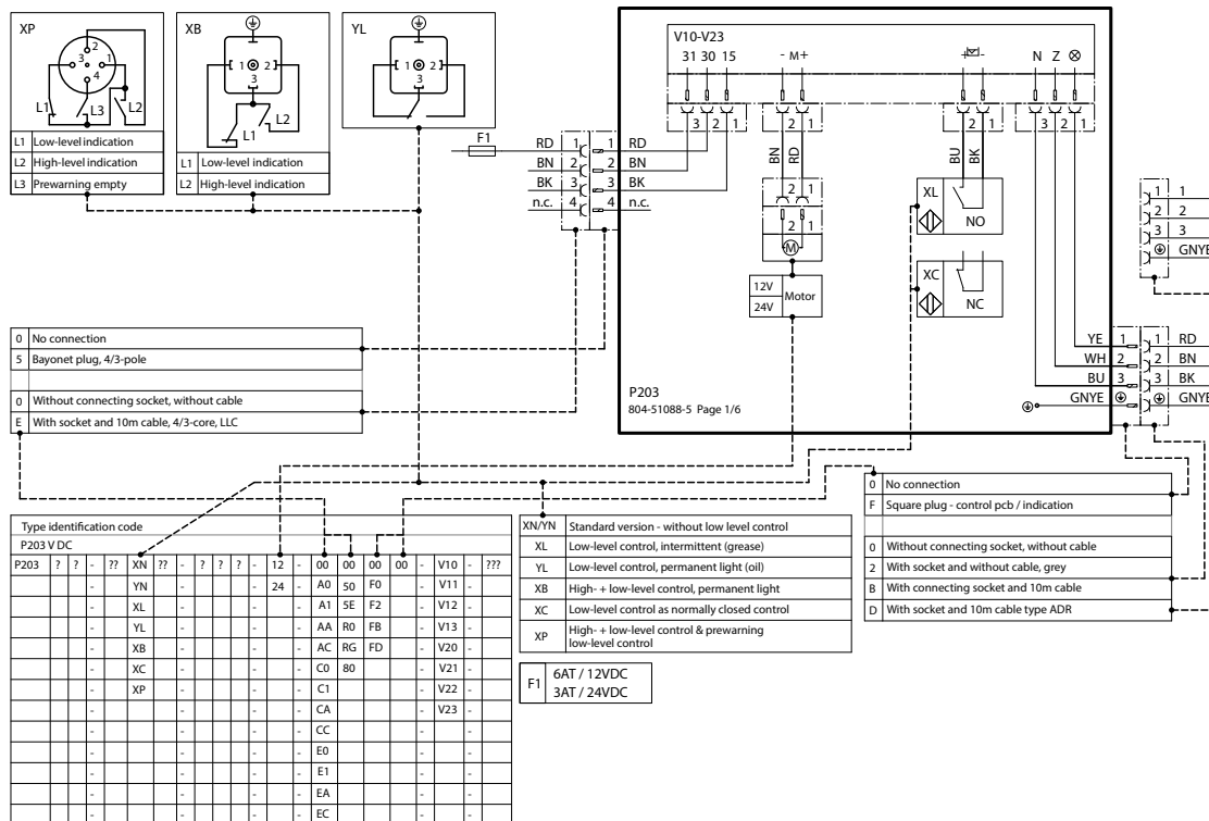
Anschlussplan P203 V DC mit Steuerplatine V Abb. 43
