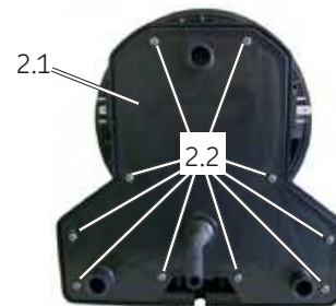
Gehäusedeckel montieren Abb. 26
