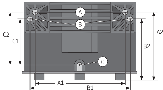
Befestigungspunkte am Pumpengehäuse der P203 Abb. 7
