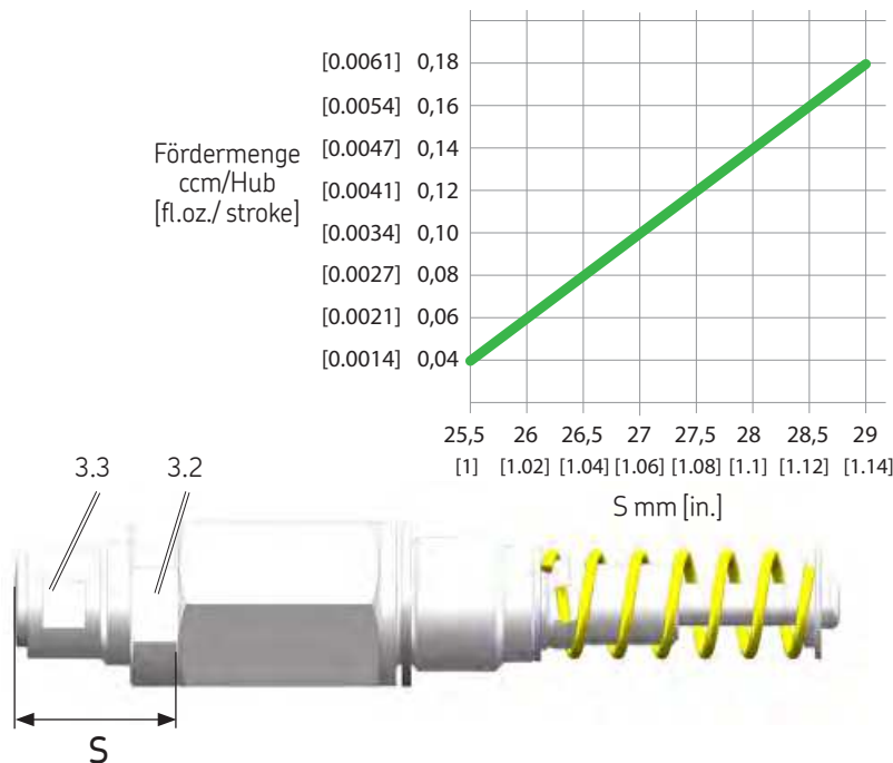
Einstellen der Fördermenge am Pumpenelement R Abb. 11
