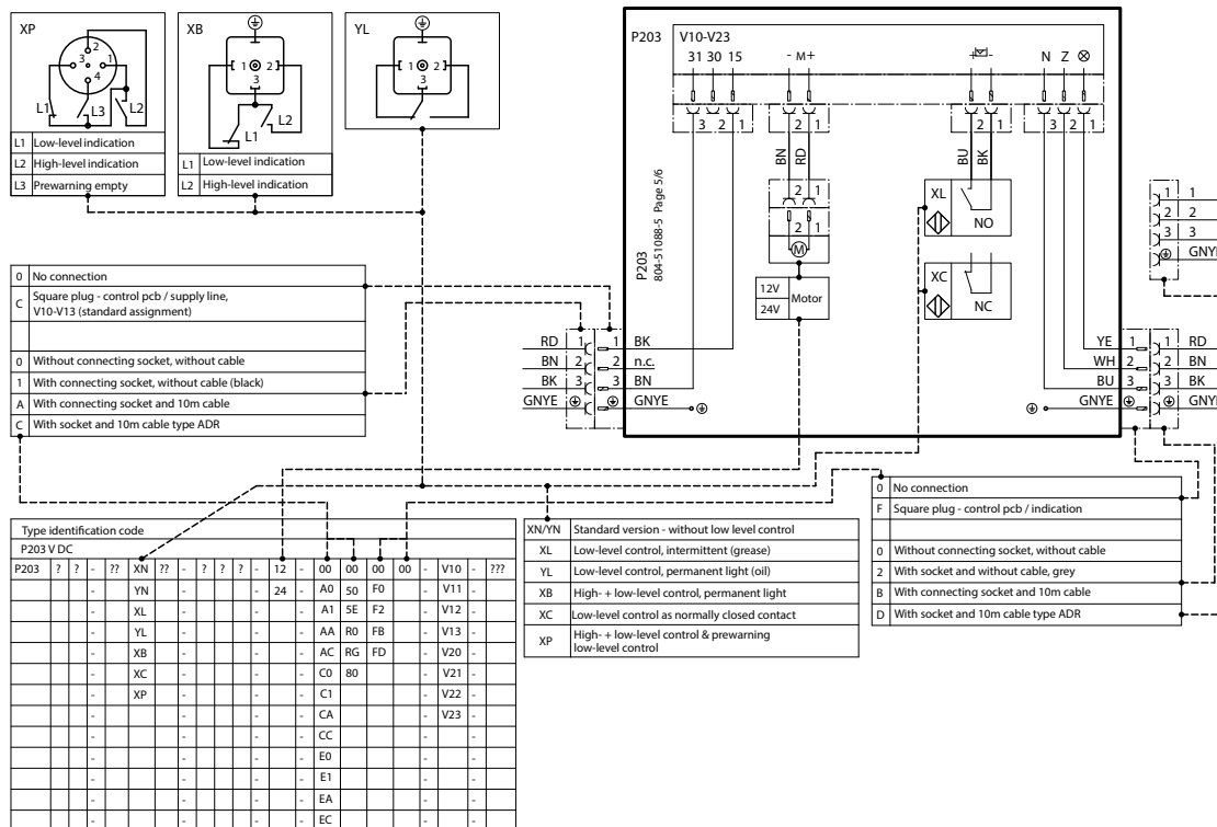
Anschlussplan P203 V DC mit Steuerplatine V Abb. 47
