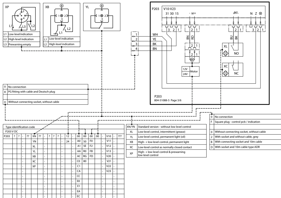
Anschlussplan P203 V DC mit Steuerplatine V Abb. 45
