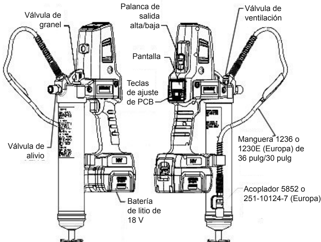
Figura 1: (pistola de engrase 1860)
